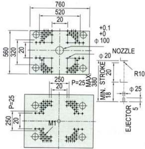
YH-75/85V
